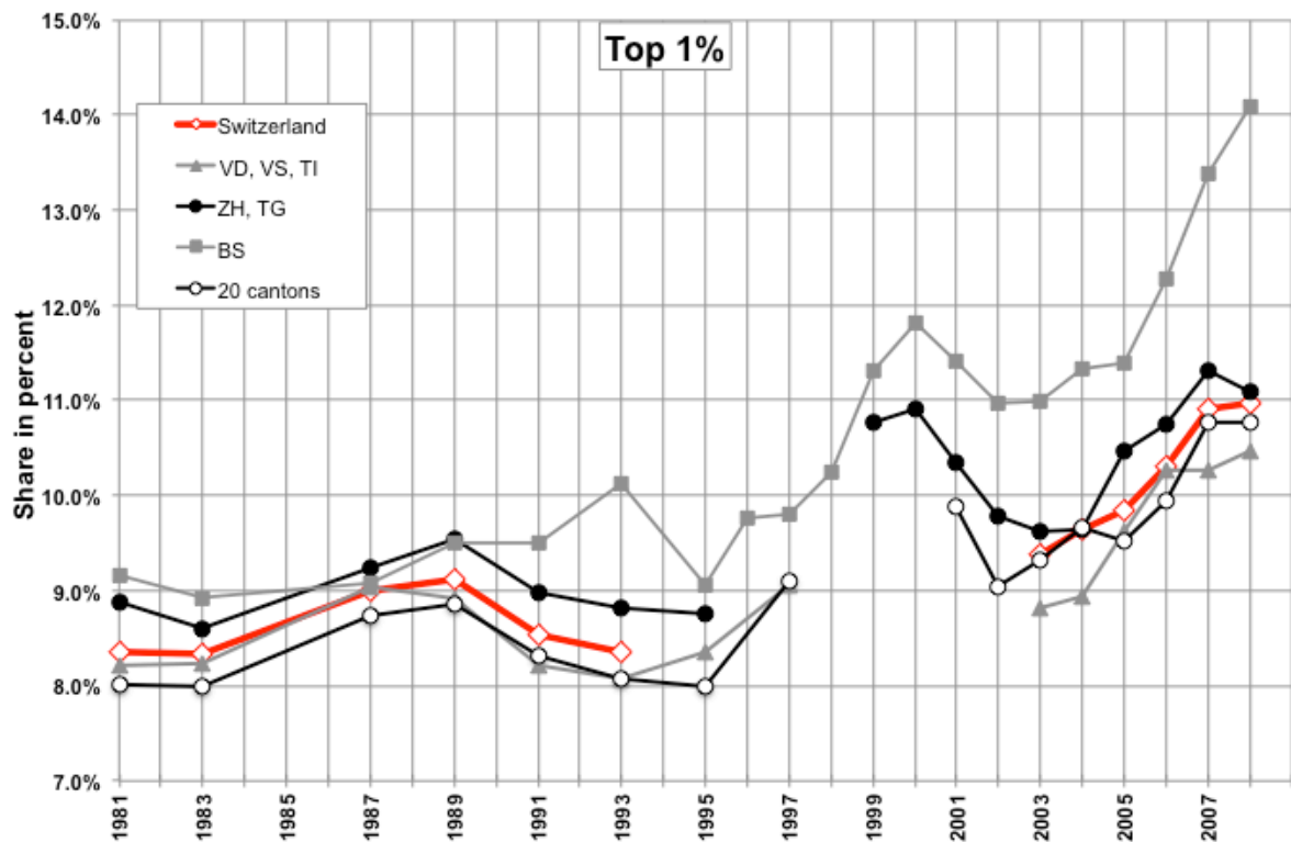
Fig. 1.c) Top 1% shares
